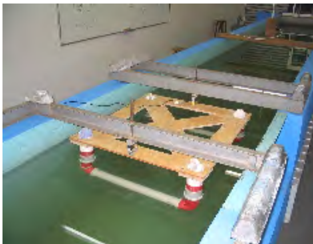
Plataforma semi-submersível sendo testada no tanque de provas do Laboratório de Engenharia Naval e Oceânica da EPUSP
